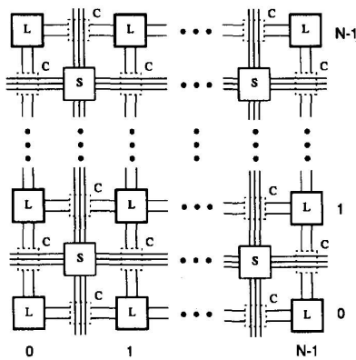
Fig. 1. An N \times N FPGA.
