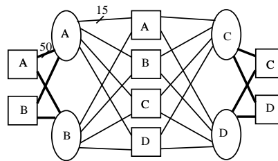
(d) Splitting Crossbars into Partial Crossbars
